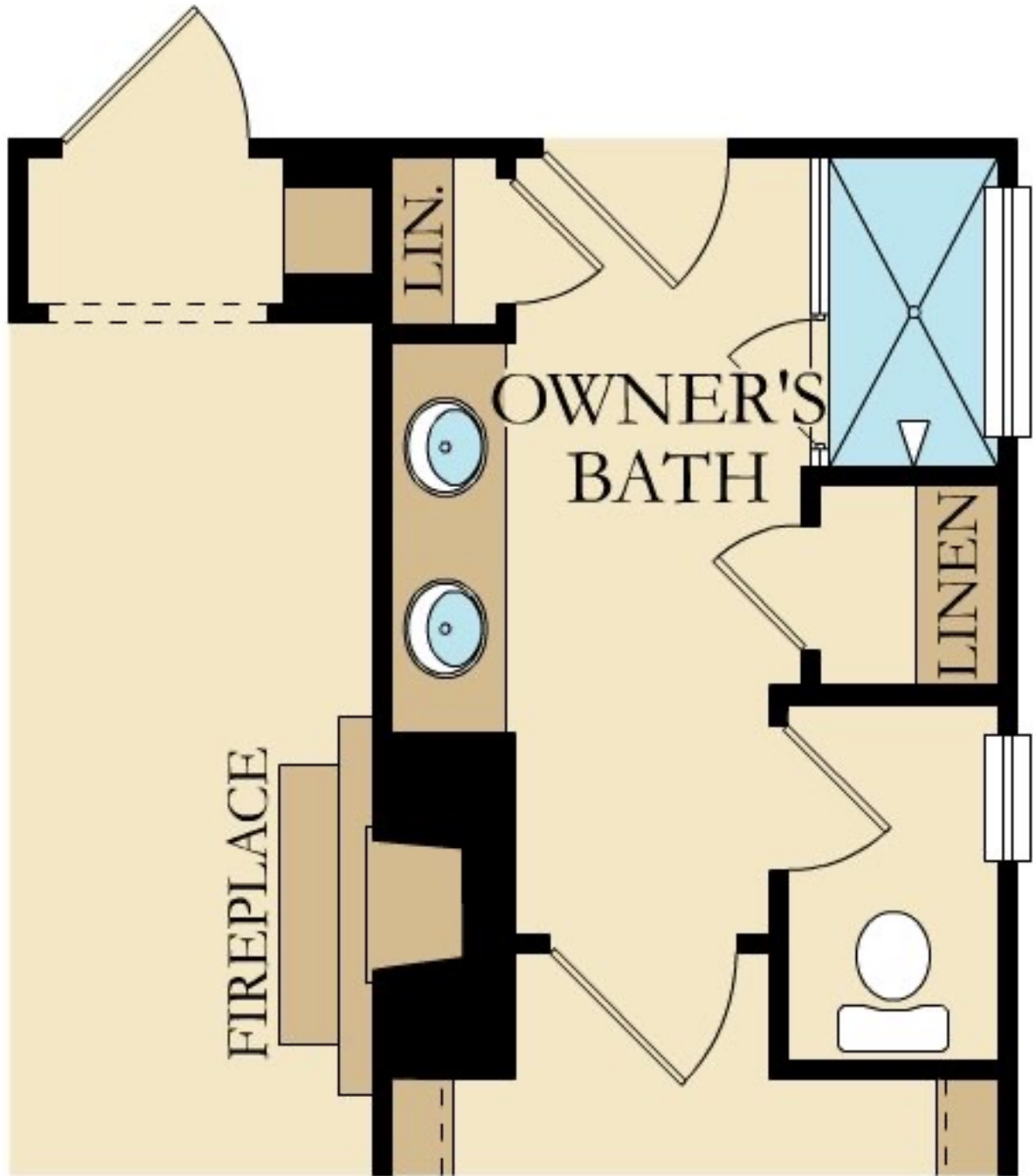
OPTIONAL FIREPLACE
